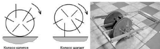
Рис.1. Принцип действия и макет шагающего колеса.
