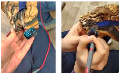
Рис. 2. Источник биометрических данных используется компактный интегральный датчик пульса/оксиметрии Maxrefdes117. Он помещен в манжет жакета.
