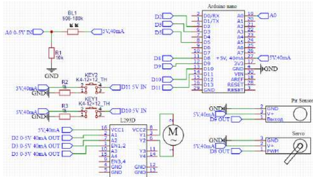
Рис. 1. Электрическая схема технического изделия
