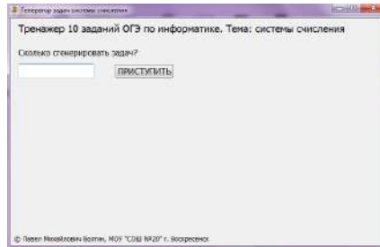
Рис. 1. Окно программы
