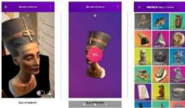
Рис. 3. Murge Cube
