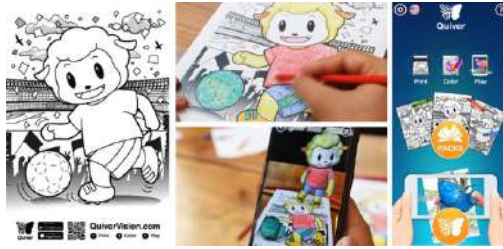
Рис. 1. Приложение Quiver
